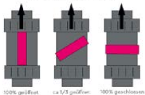
Kugelhahnstellung
